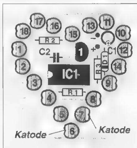
Figuur 2: De componentenopstelling.
